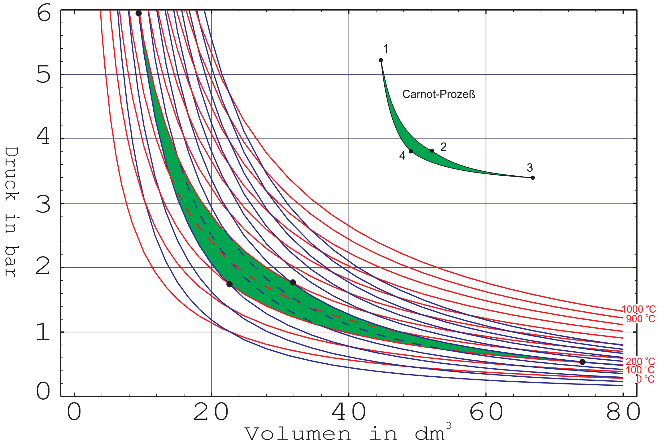
pV-Diagramm der Isothermen und Adiabaten von 1 mol des Idealen Gases
